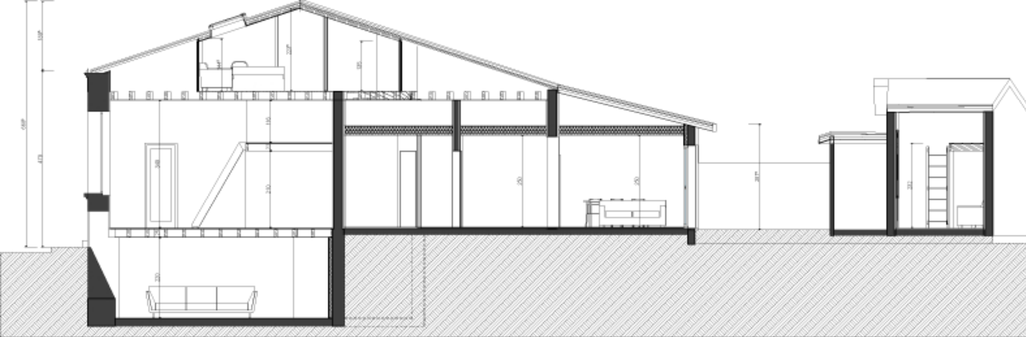
COUPE AA
